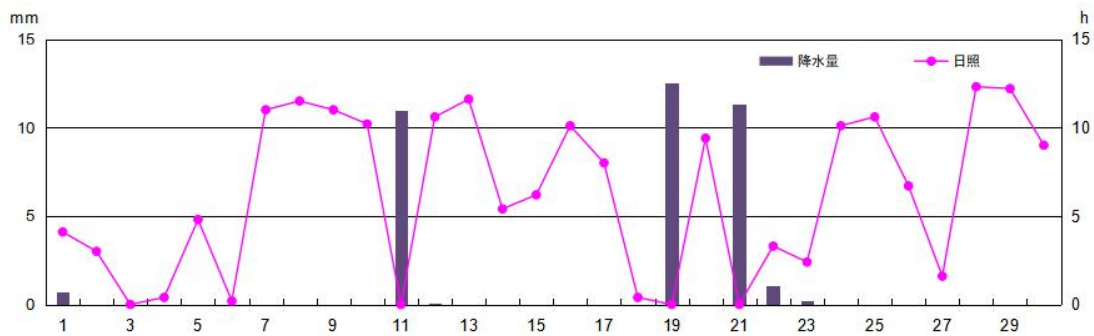
2020 年 4 月鄞州国家基本气象站日降水量和日照时数变化图
