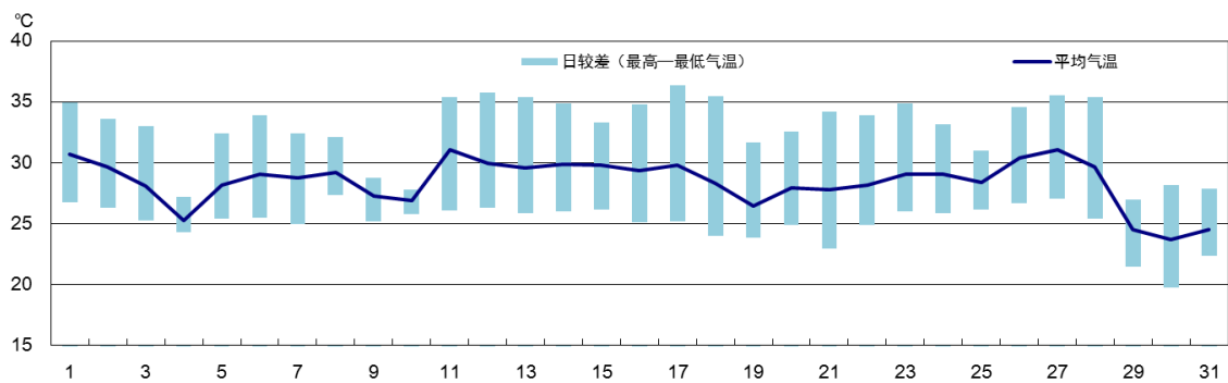
2019 年 8 月鄞州国家基本气象站日平均气温和气温日较差变化图
