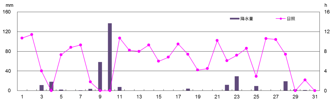
2019年8月鄞州国家基本气象站日降水量和日照时数变化图
